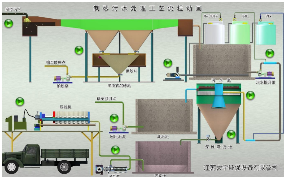
图 8.3-1 本项目废水处理工艺流程图
