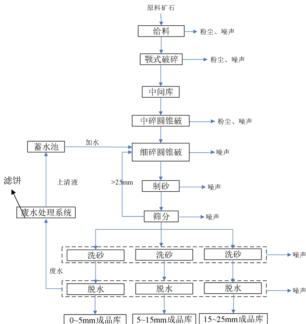
图 3.1-5 矿石加工工艺流程及产污节点示意图
