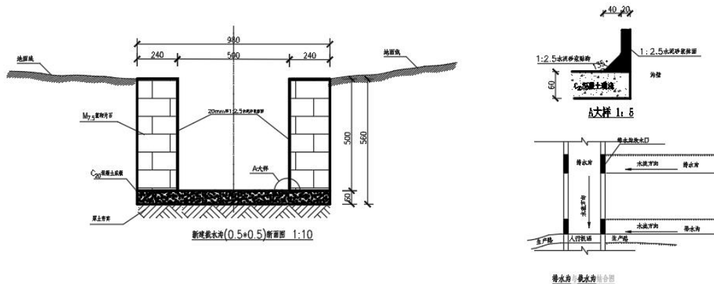
图 8.1-1 工业广场截水沟典型设计图
