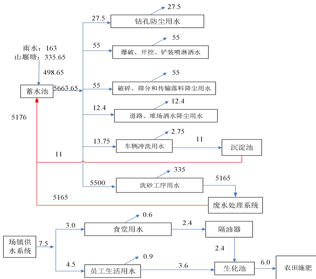
图 3.2-1 项目水平衡图 (m 3 /d)
