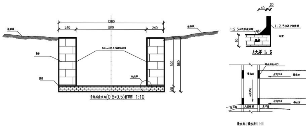
图 8.1-3 采坑底部排水沟典型设计图
