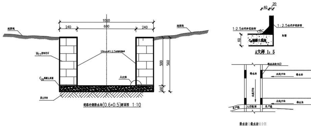
图 8.1-2 道路内侧排水沟典型设计图
