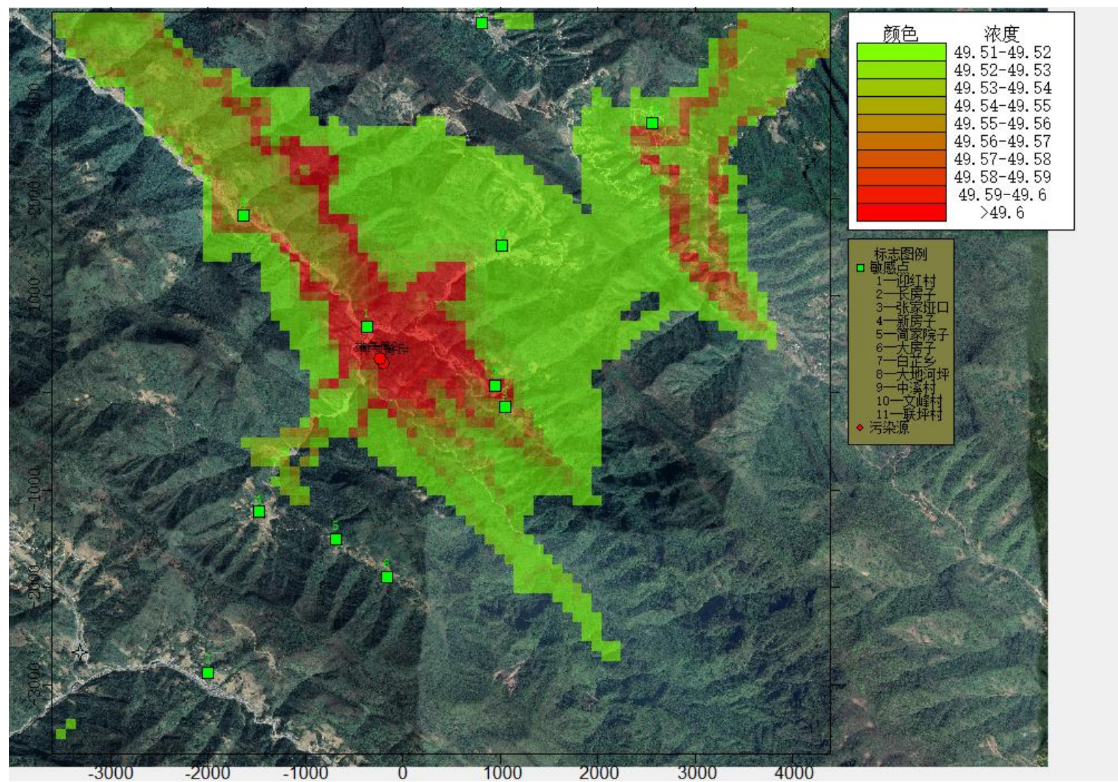
图 6.2-2 PM 10 叠加现状后年均浓度分布图
