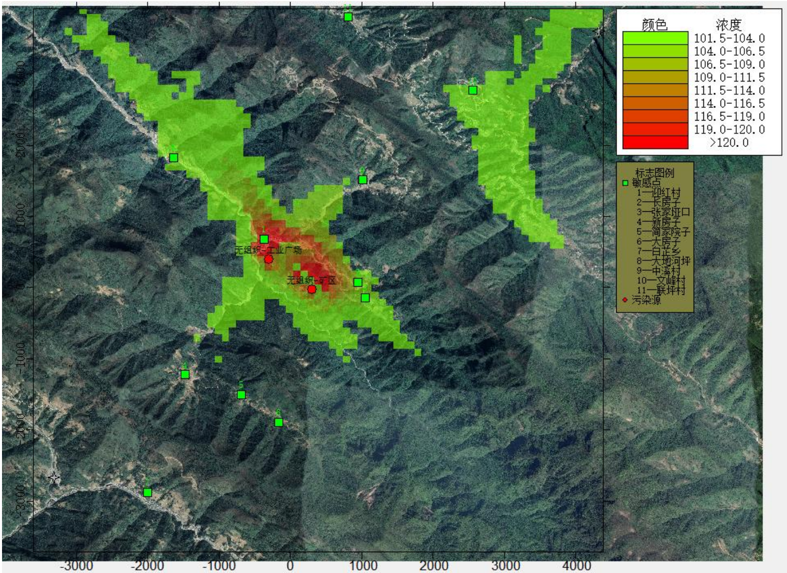
图 6.2-3 TSP 叠加现状后年均浓度分布图
