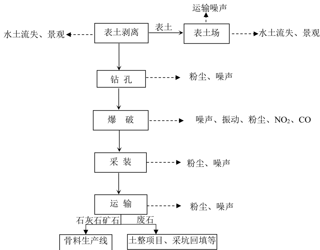
图 3.1-4 开采工艺流程及产污节点示意图
