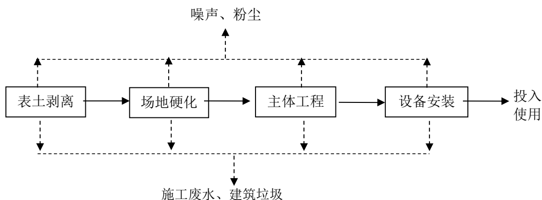
图 3.1-2 工业广场建设期施工工艺及产排污环节图
