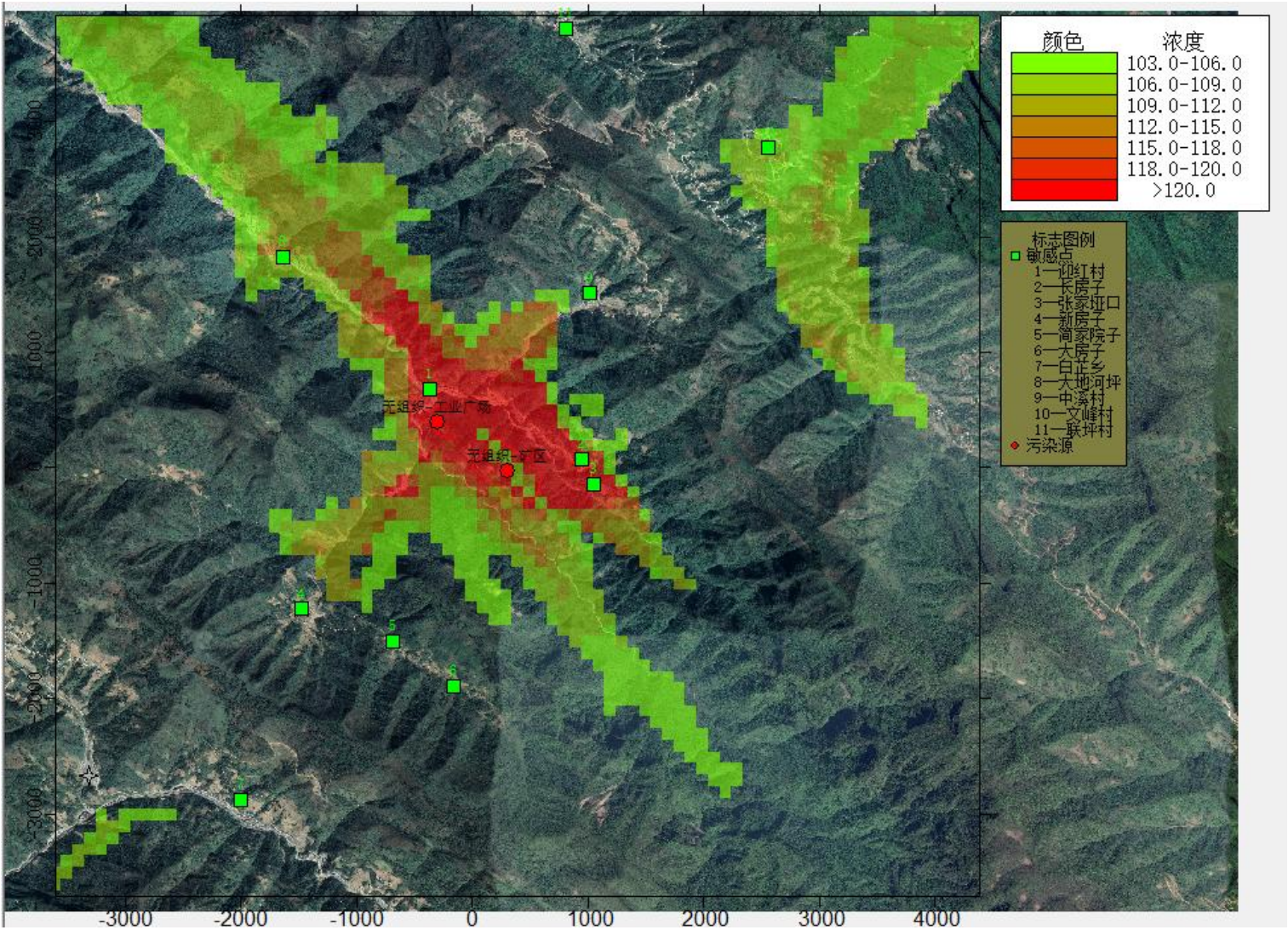
图 6.2-3 TSP 叠加现状后日均浓度分布图
