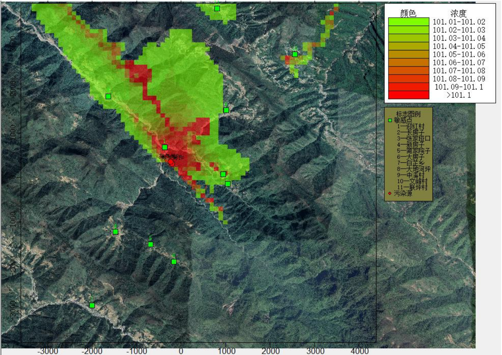
图 6.2-1 PM 10 叠加现状后 95%保证率日平均质量浓度分布图
